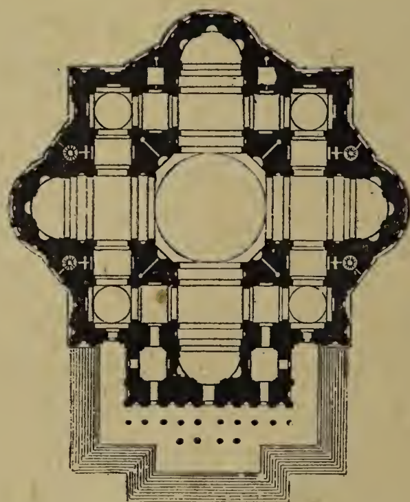
FIGURA 309—(Springer, o. c. ). Planta para la basílica de S. Pedro Vaticano, según la refundición de Miguel Angel
